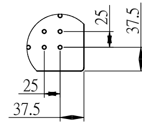
細部放大圖 A 比例 1:6
