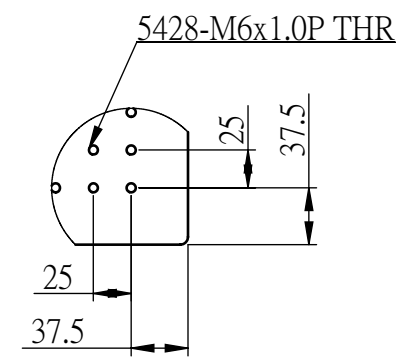
細部放大圖 A 比例 1:5
